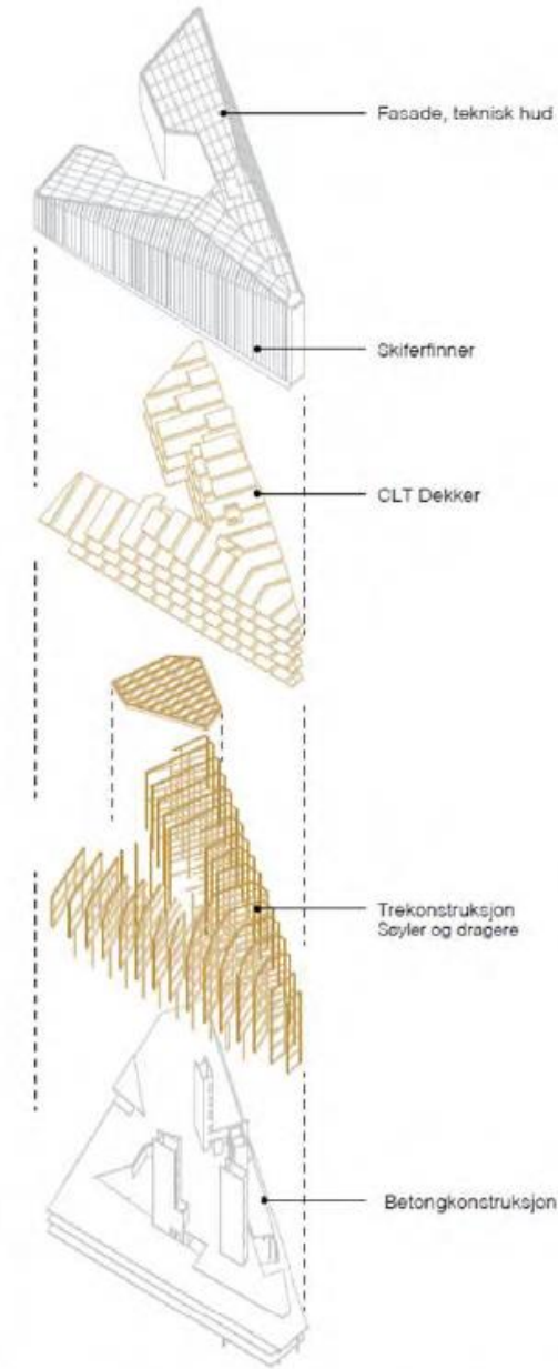
Eksploderte aksonometri av konstruksjonselementer
